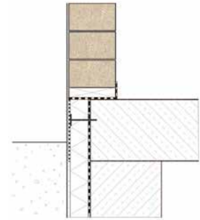
Anschluss gedämmter Keller
